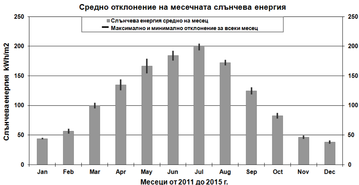
Фиг. 4. Средно измерена слънчева енергия за всеки месец
