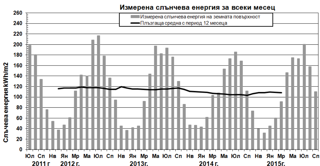
Фиг. 5. Плъзгаща се центрирана математическа средна на слънчева енергия по 12 месеца
