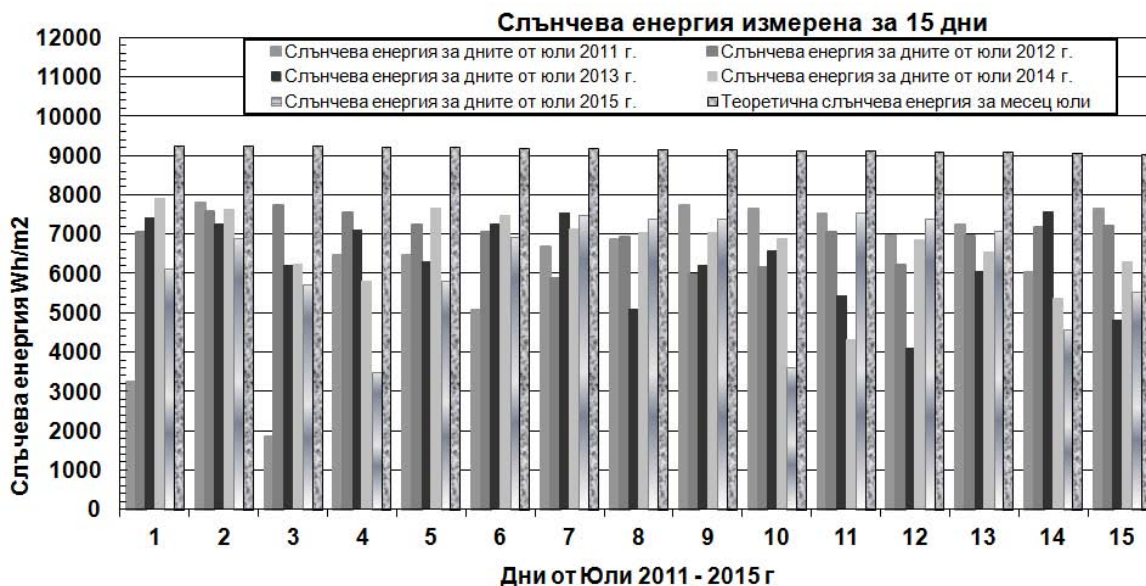
Фиг. 1. Слънчева енергия измерена за всеки ден от 1 до 15 юли от 2011 до 2015 година
